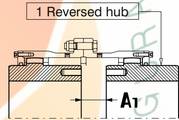
Fig. 41 - SID-R Coupling
