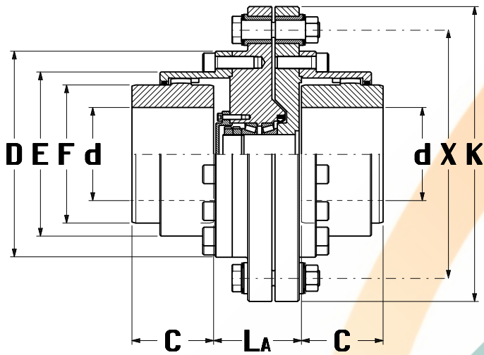
Fig. 30 - GO-AS Coupling
