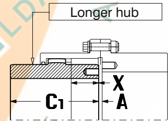
Fig. 10 - GO-FAM Coupling
