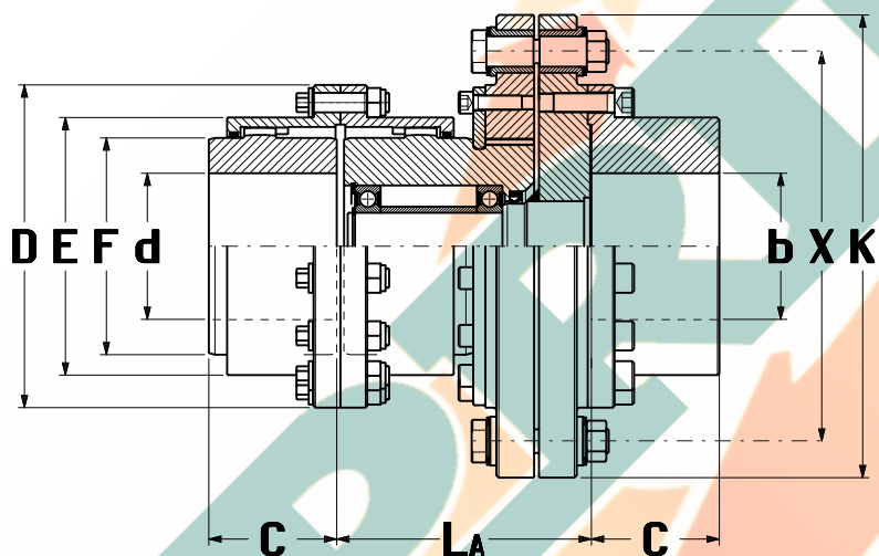
Fig. 33 - GO-ASX Coupling
