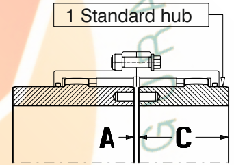
Fig. 06 - GO-AM Coupling
