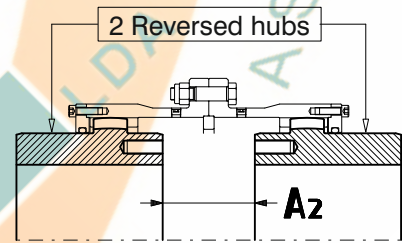
Fig. 42 - SID-RR Coupling
