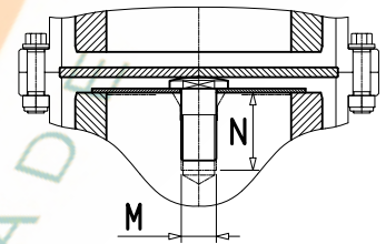
Fig. 17 AO-AV Spacer Couplings
